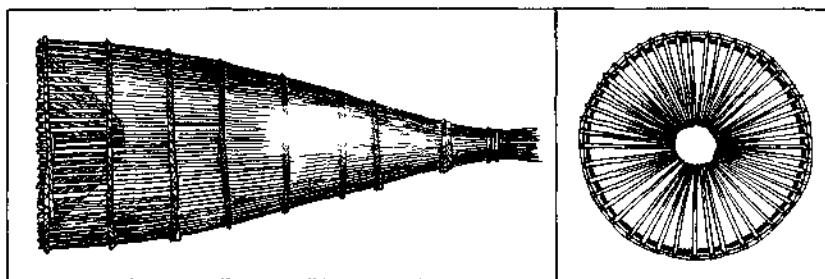
figuur 7 fuik (zyaanzicht en vooraanzicht, schaal 1:18)
