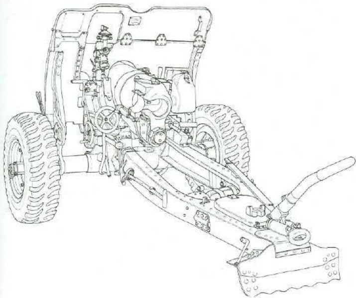
De Britse 4.5-inch houwitser. Lengte loop: 13,33 maal het kaliber. Gewicht granaat: 15,75 kg. Maximale dracht: ongeveer 6400 m. Elevatiehoek: -5° tot +45°. Gewicht van kanon met affuit: ongeveer 1350 kg.
